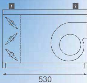
1. Многостворчатый клапан. 2. Вентилятор
