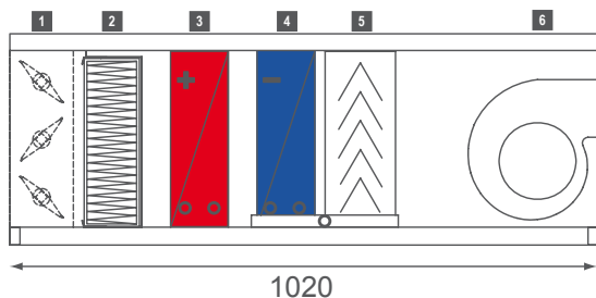
1. Многостворчатый клапан. 2. Воздушный фильтр. 3. Водяной воздухонагреватель. 4. Воздухоохладитель. 5. Каплеотделитель. 6. Вентилятор.
