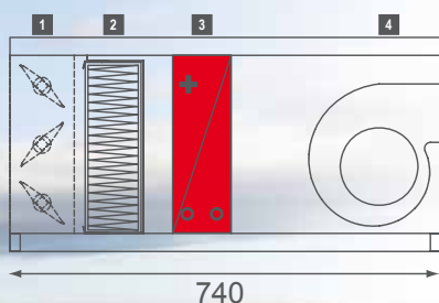
1. Многостворчатый клапан. 2. Воздушный фильтр. 3. Водяной воздухонагреватель. 4. Вентилятор.
