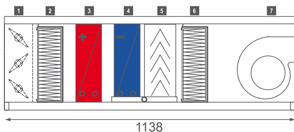
1. Многостворчатый клапан. 2. Воздушный фильтр F5. 3. Водяной воздухонагреватель. 4. Воздухоохладитель. 5. Каплеотделитель. 6. Воздушный фильтр F7. 7. Вентилятор.
