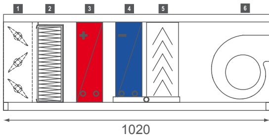
1. Многостворчатый клапан. 2. Воздушный фильтр. 3. Водяной воздухонагреватель. 4. Воздухоохладитель. 5. Каплеотделитель. 6. Вентилятор.
